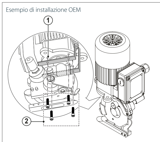
Schema di fissaggio per installazione OEM
