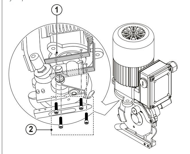
Ejemplo de instalación OEM
