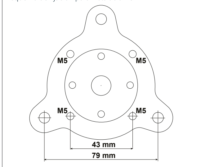
Esquema de fijación para instalación OEM
